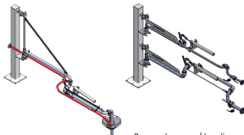
Brazos de carga / Loading arms
